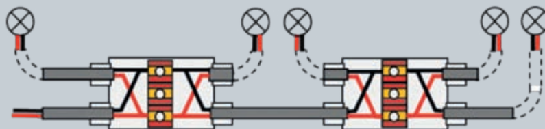
Vzporedni priključni sistem s petimi svetilkami
